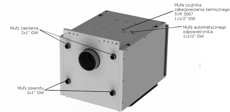
Widok kotła bez kosza z tyłu
