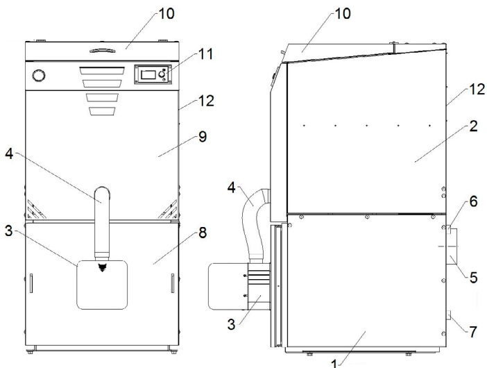
Rys.4. Kocioł „SlimKo Plus”
