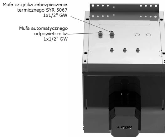
Widok kotła bez kosza z przodu
